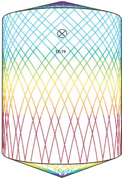
D8m H10m, Toftejorg MJ50, 4 x ø10mm 0 % Tiempo = 5.5 mín., Consumo de agua = 2565 l
