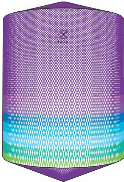
D8m H10m, Toftejorg MJ50, 4 x ø10 mm, 0 % Tiempo = 23.3 mín., Consumo de agua = 10868 l
